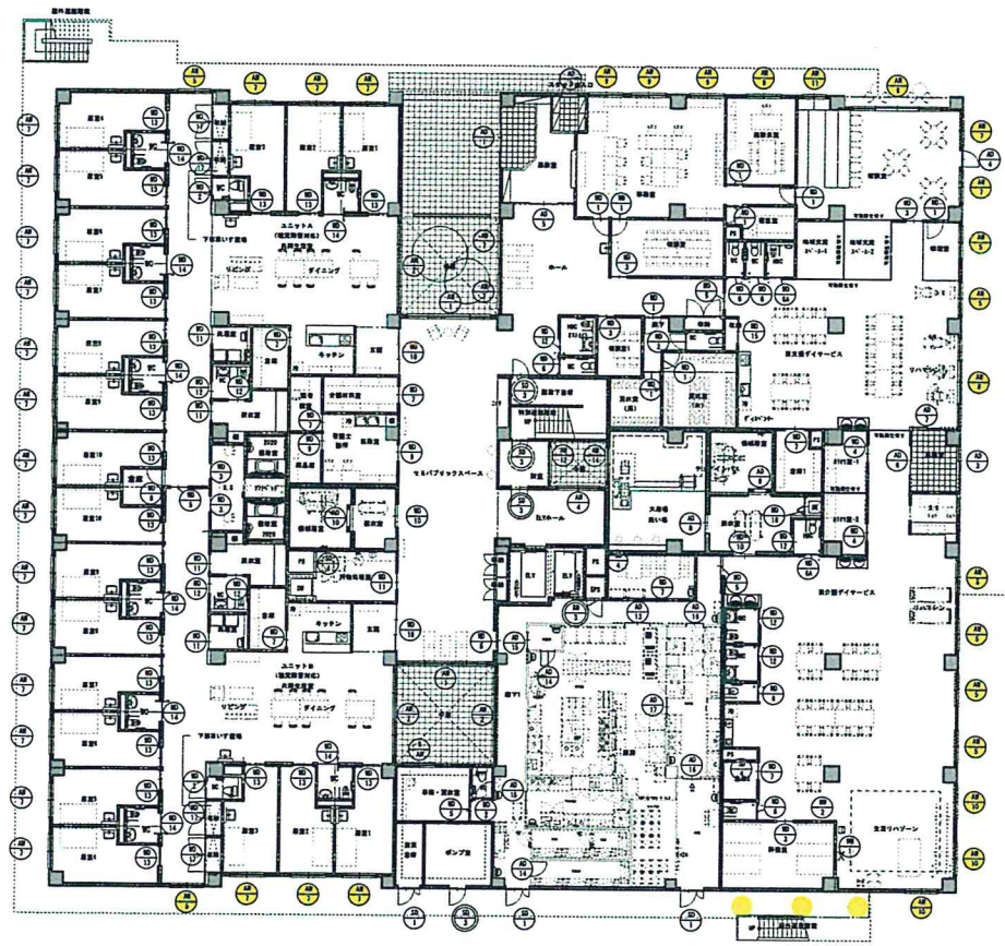
1階器具配置図 S=1:150
