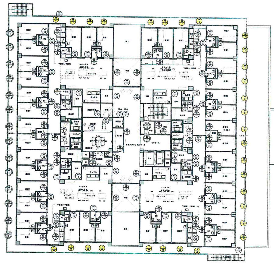
2階器具配置図 S=1:150
